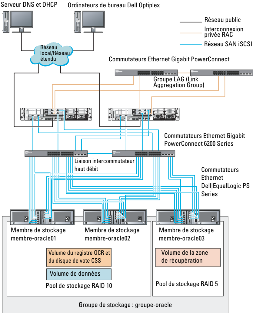
Figure 6-2. Configuration d'un cluster Oracle RAC fictif à trois matrices PS6000XV
