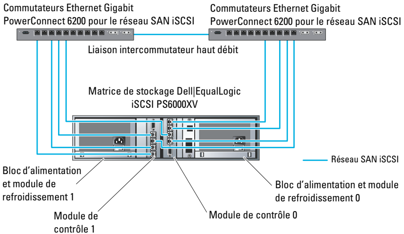
Figure 6-1. Configuration réseau recommandée
