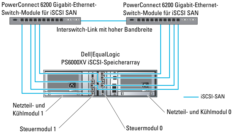
Abbildung 6-1. Empfohlene Netzwerkkonfiguration
