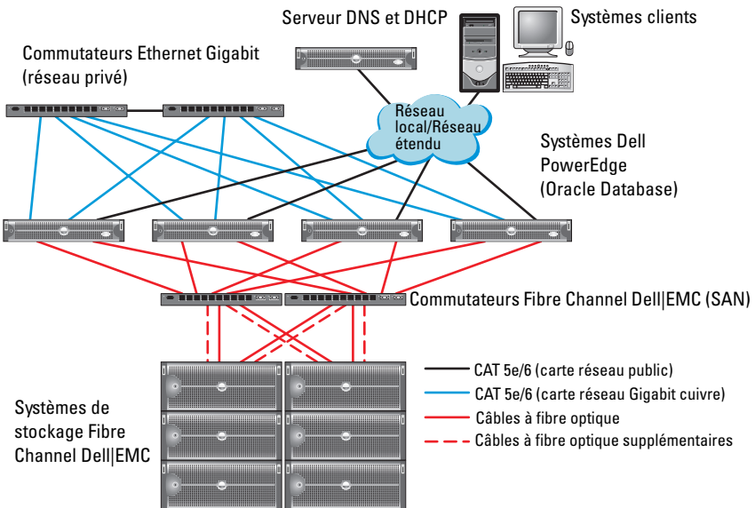
Figure 3-1. Connexions matérielles pour un cluster Fibre Channel
