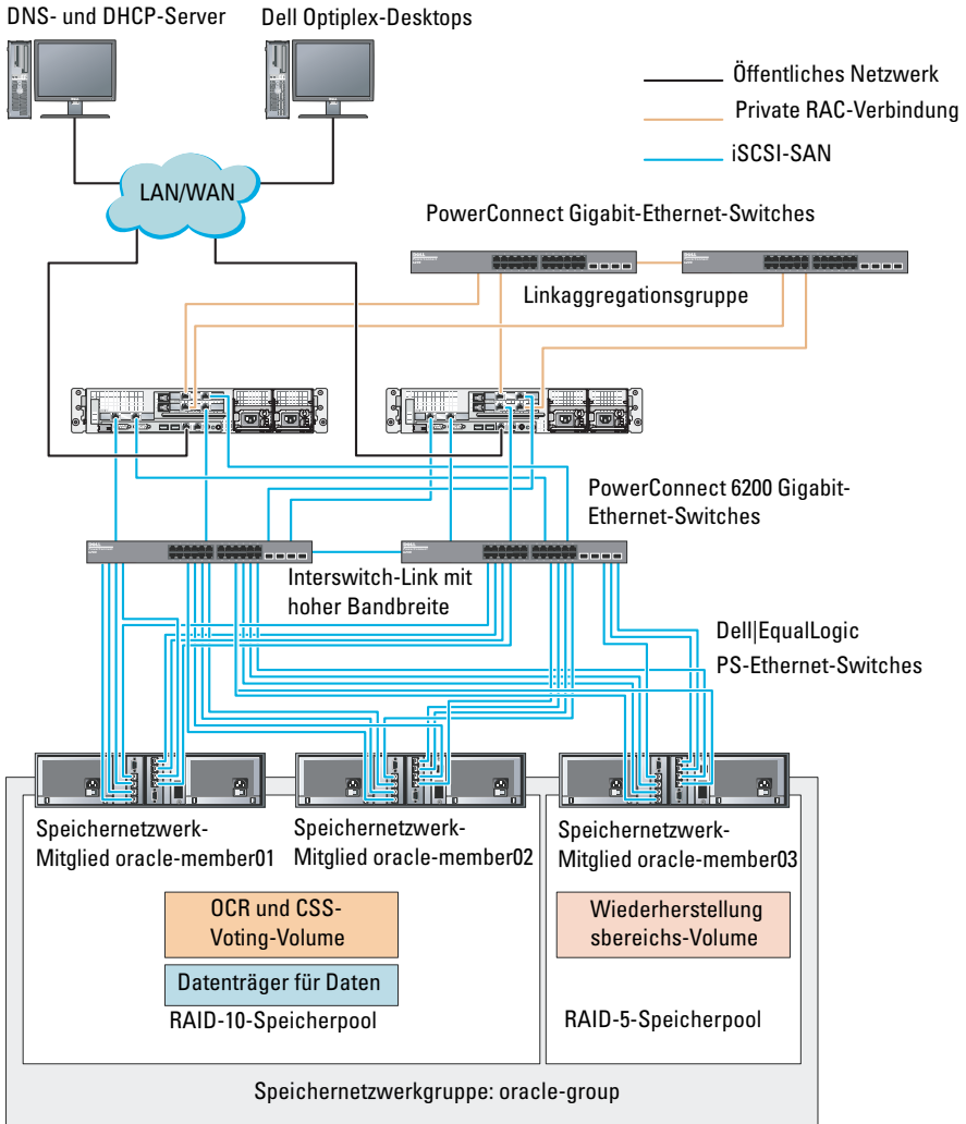
Abbildung 6-2. Beispielkonfiguration eines Oracle RAC mit drei PS6000XV-Arrays
