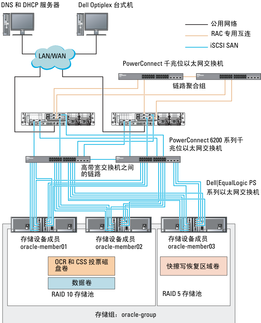
图 6-2. 配置带有三个 PS6000XV 阵列的示例 Oracle RAC
