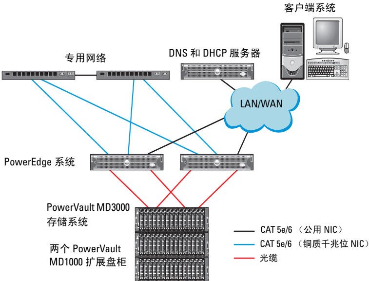
图 4-1. 串行连接的 SCSI (SAS) 群集和 Dell PowerVault MD3000 存储设备盘柜布线
