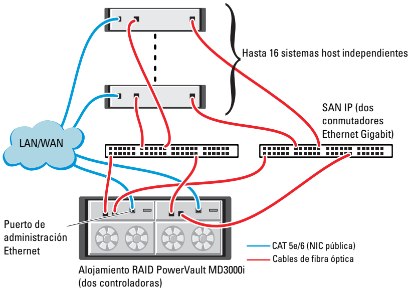
Ilustración 5-2. Cableado de los clústeres iSCSI conmutados
