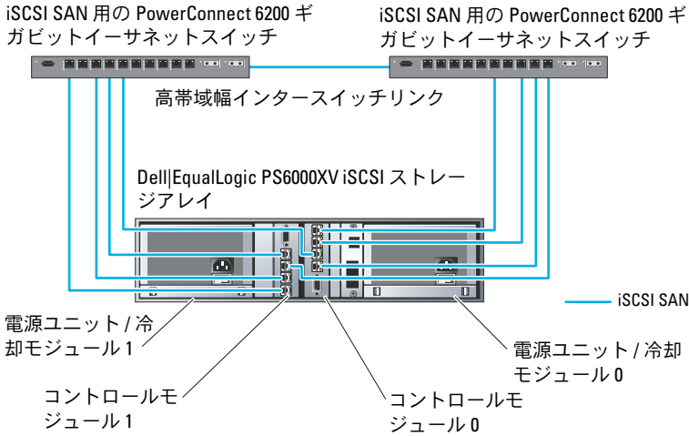
図 6-1 推奨ネットワーク構成
