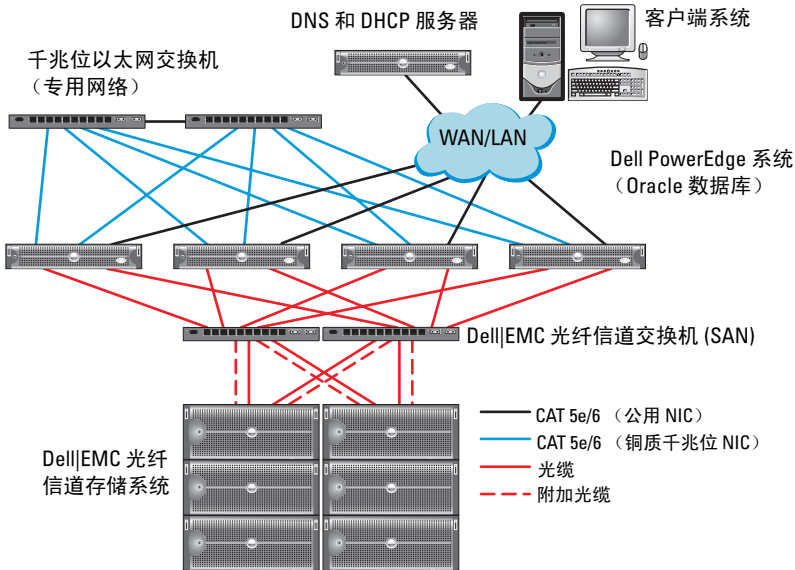
图 3-1. 光纤信道群集的硬件连接
