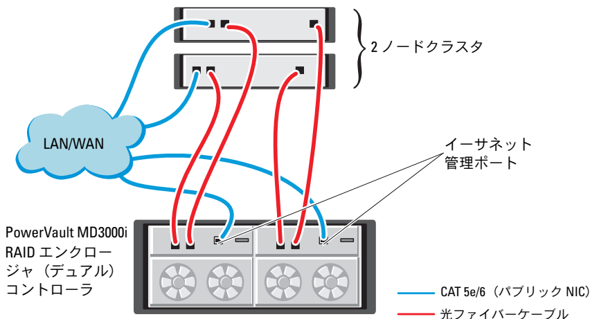
図 5-1 iSCSI 直接接続クラスタのケーブル接続
