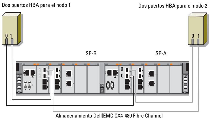
Ilustración 3-2. Cableado de un clúster Fibre Channel de conexión directa
