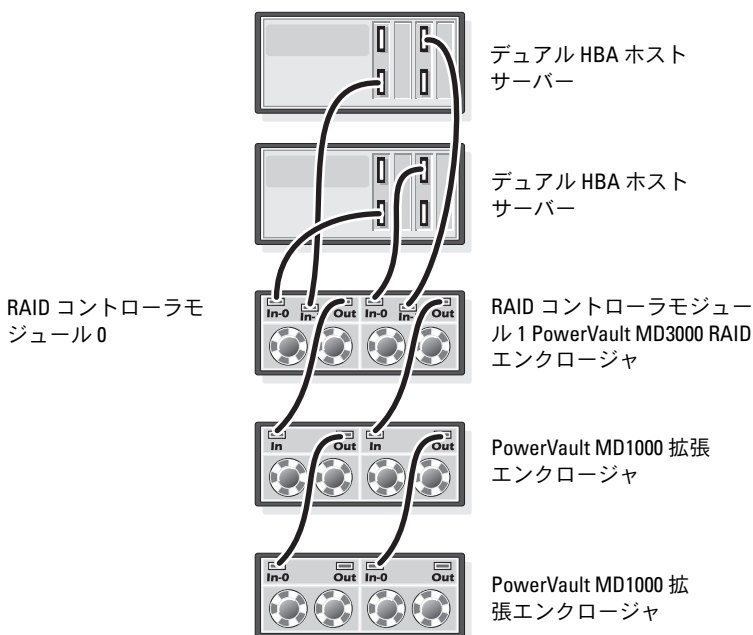
図 4-2 直接接続 SAS クラスターのケーブル接続
