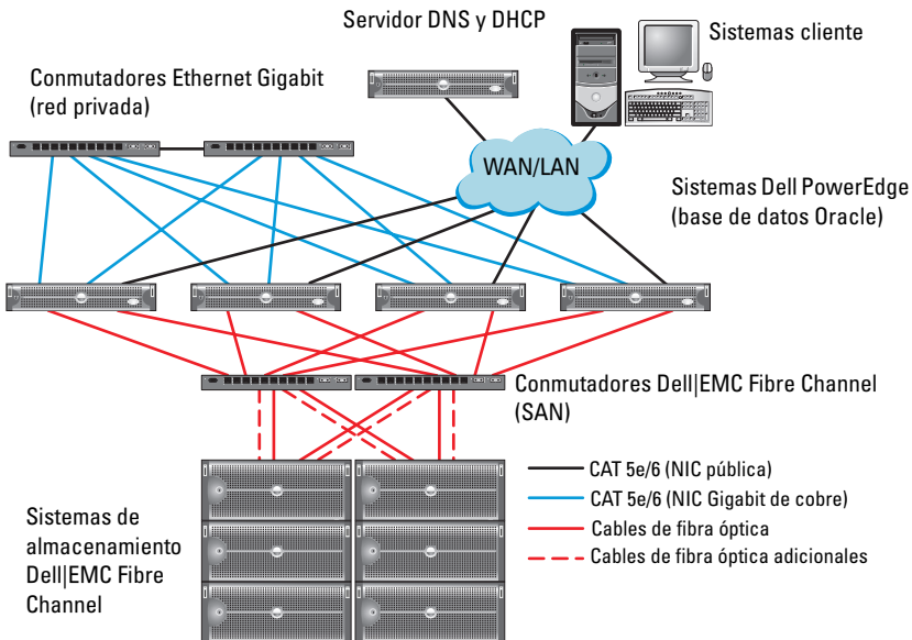
Ilustración 3-1. Conexiones de hardware para un clúster Fibre Channel
