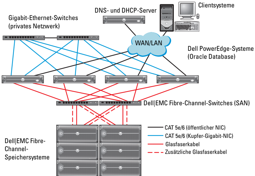
Abbildung 3-1. Hardwareverbindungen für einen Fibre-Channel-Cluster
