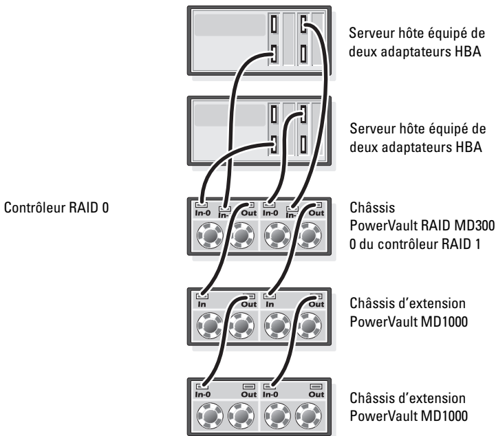
Figure 4-2. Câblage d'un cluster SAS à connexion directe
